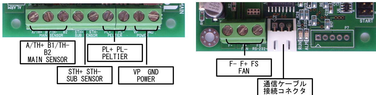
接続端子の配置
