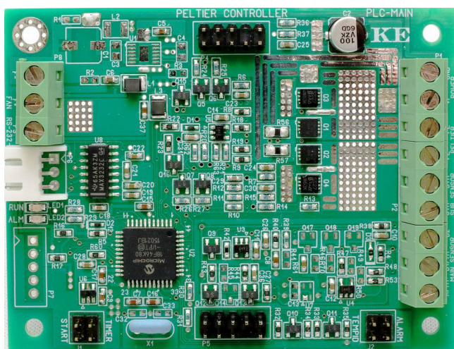
本体基板外観
